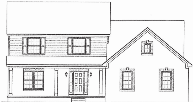
ELEVATION - B
